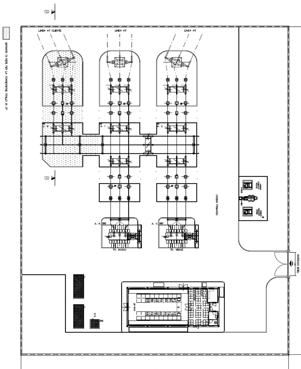
Figura E-1: Impianto di rete per la connessione stallo in Cabina Primaria per Cliente Passivo distante da Cabina Primaria (Vista in pianta).
