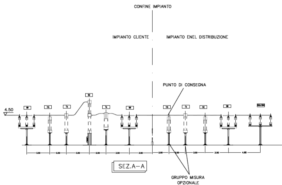
Figura E-13: Allacciamento Cliente AT Attivo in antenna su stallo di Cabina Primaria impianto adiacente alla Cabina Primaria (Vista laterale).
